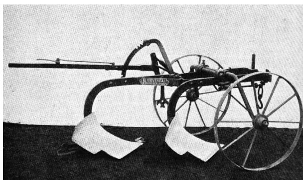
Arado de asiento El Universal, diseñado y fabricado por Nicolás Schneider en la década de 1870. Fuente: Miatello, H., o. cit., p. 482
